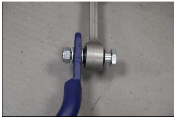
Abb. 2: Schraube mit ca. 50 Nm anziehen.
